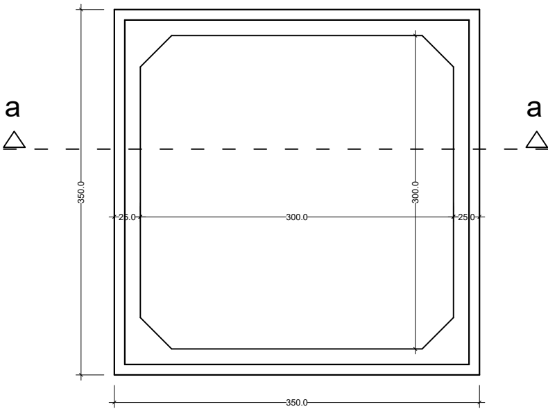
Tombina betonarme me dim. 300x300x200 cm'
